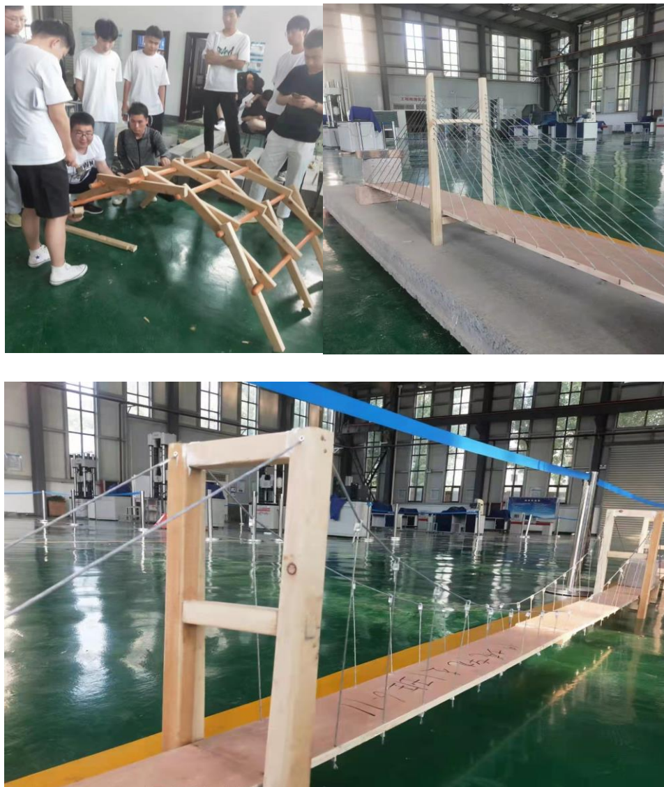
图3 桥梁微模型
